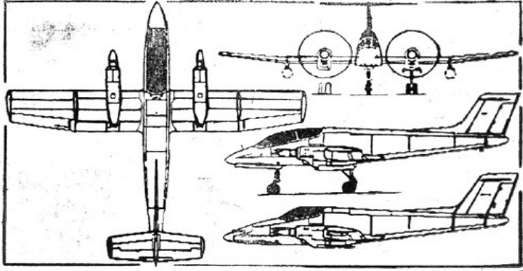
'புக்காரா' ரகத்தைச் சேர்ந்த - ஐ. ஏ. 58 ஏ வகை வானூர்தியினதும் (இரு இருக்கைகள் கொண்டது - பக்கப் பார்வையில் மேலே உள்ளது), ஐ. ஏ. 58 சி வகை வானூர்தியினதும் (ஒரு இருக்கை கொண்டது - பக்கப் பார்வையில் கீழே உள்ளது) மாதிரித் தோற்றங்கள்.
